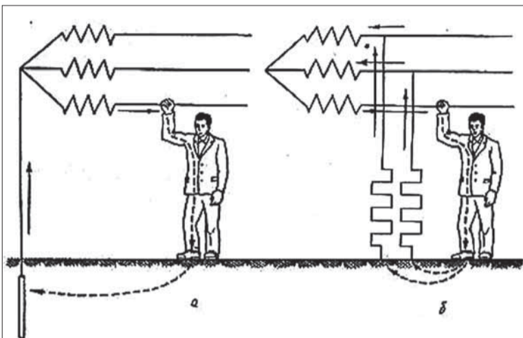
Рис. 2. Однофазное включение в цепь тока: а) с заземленной нейтралью; б) с изолированной нейтралью
